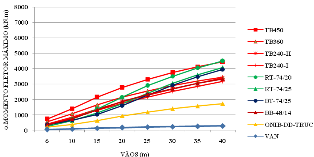
Figura 5.5 – Comparação dos efeitos dos carregamentos, excluindo carga permanente, com os respectivos coeficientes de impacto. Veículos atuando em faixa simples
