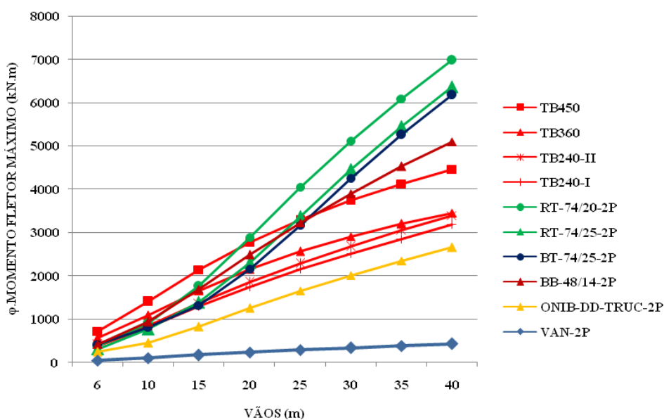
Figura 5.6 – Comparação dos efeitos dos carregamentos, excluindo carga permanente, com os respectivos coeficientes de impacto. Veículos atuando em duas faixas
