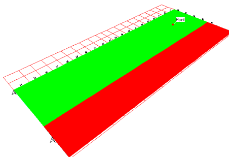
Figura 4.3 – Faixas de atuação do TB360 e TB450, multidão (verde) e veículo (vermelho)
