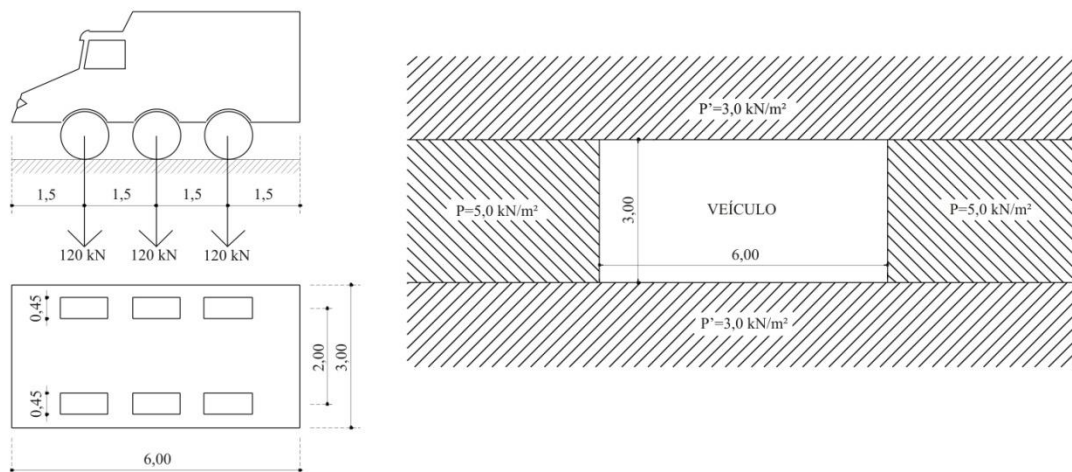
Figura 2.3 – Esquema de carregamento da NB-6/1960
