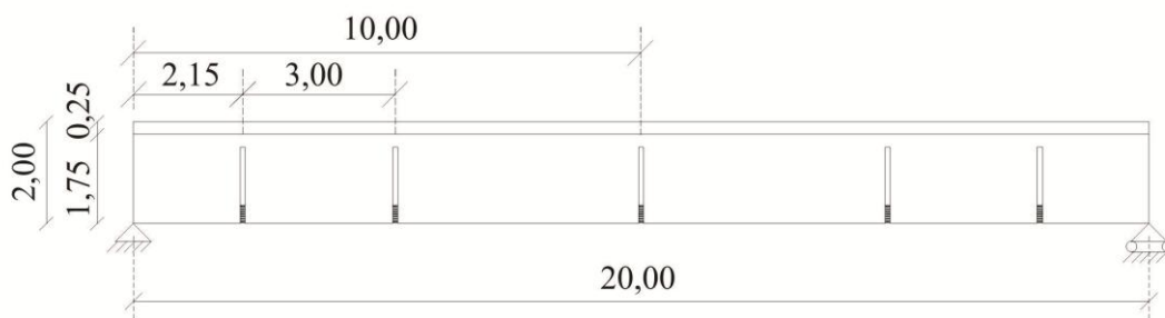
Figura 7 – Longarina com cinco fissuras de 1,50m (5F150)
