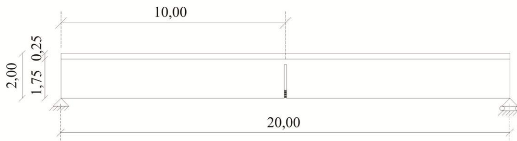
Figura 6 – Longarina com uma fissura de 1,50m no meio do vão (F150)
