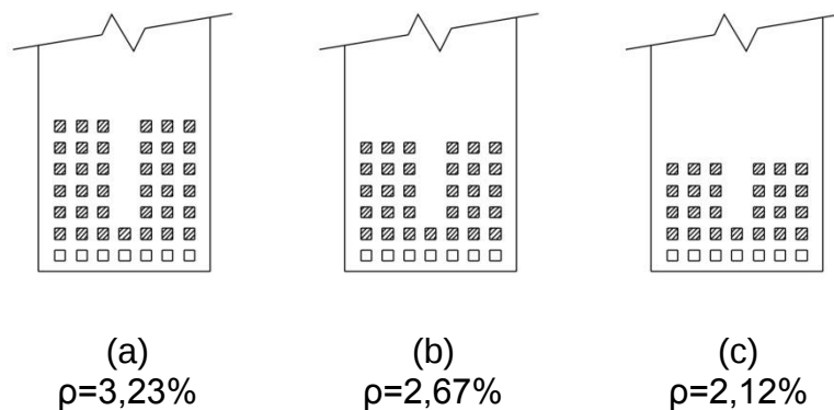
Figura 5 – Distribuição das barras na seção transversal das longarinas, com a primeira camada com 100% de corrosão (MENDES (2009))
