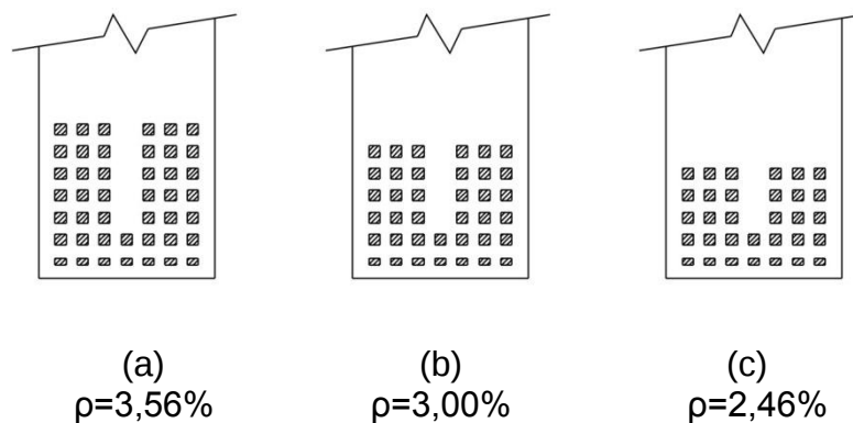
Figura 4 – Distribuição das barras na seção transversal das longarinas, com a primeira camada com 40% de corrosão (MENDES (2009))
