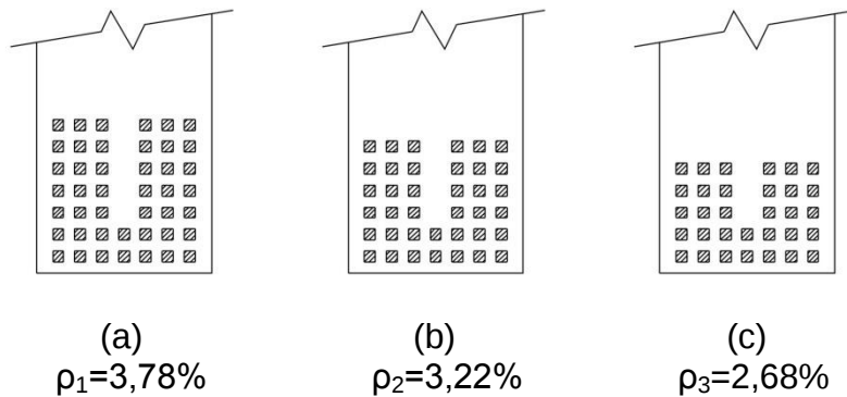
Figura 3 – Distribuição das barras na seção transversal das longarinas (MENDES (2009))
